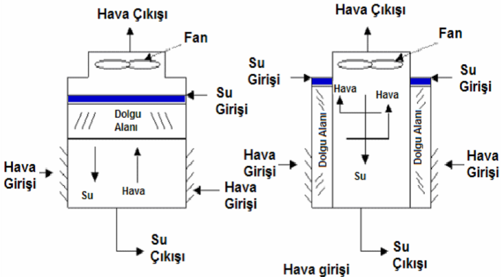
Şekil 3. Karşı ve Çapraz Akışlı Kule Tasarımı
